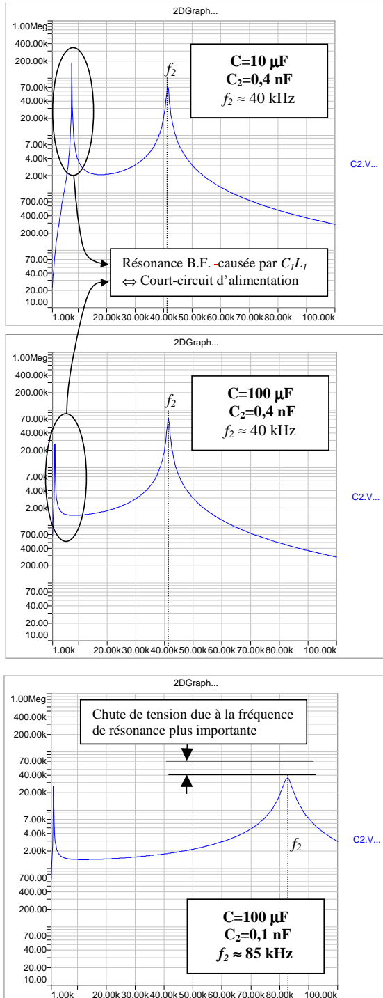
Fig 9 : Simulations sous Simplorer [4]
