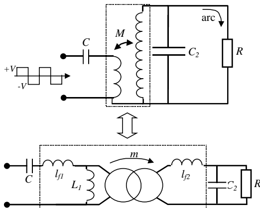
Fig 6 : Modélisation du transformateur équivalent
