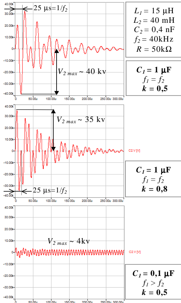
Fig 3 : Simulations sous Simplorer [4]
