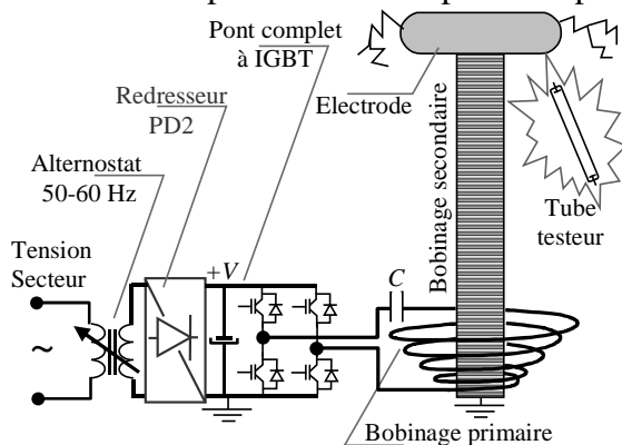
Fig 5 : Alimentation en créneaux à f réglable
