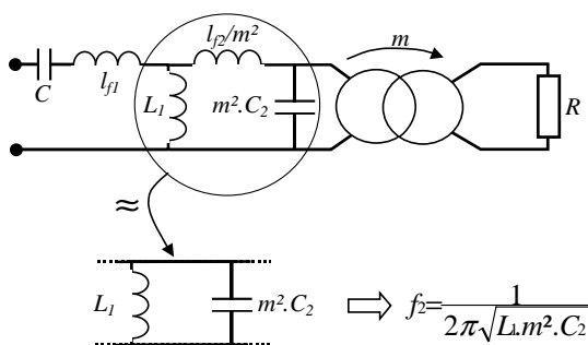
Fig 7 : Manipulation du modèle
