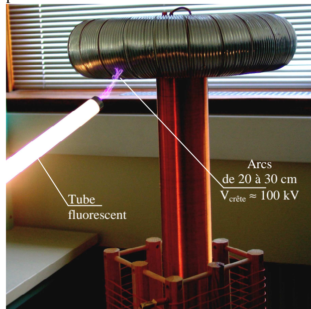
Fig 10 : Bobine et effluves attirées par un tube néon
