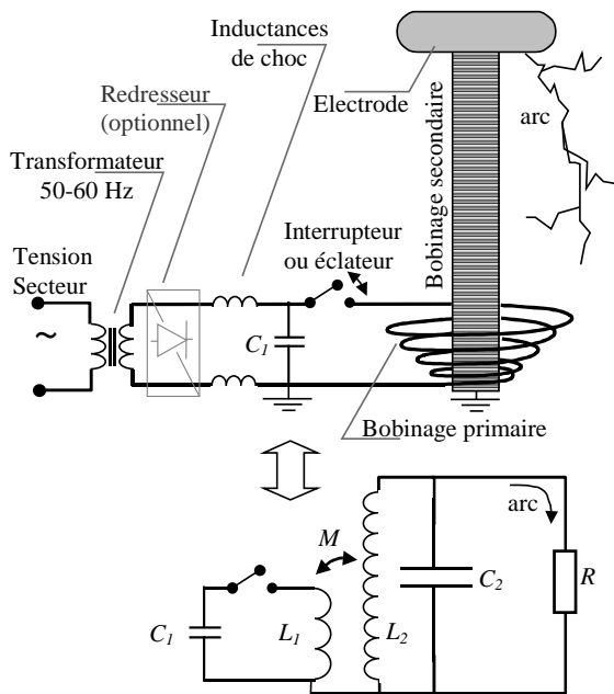
Fig 2 : Alimentation « en lâché » et modèle électrique
